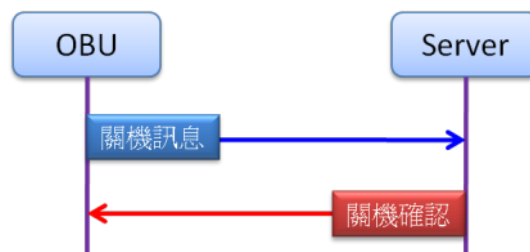
圖 3-9 關機回報流程
