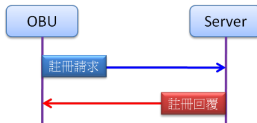
圖 3-4 註冊流程
